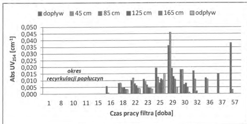
Rys. 9. Zmiana absorbancji UV254 w przekroju filtra 2 w czasie jego eksploatacji
