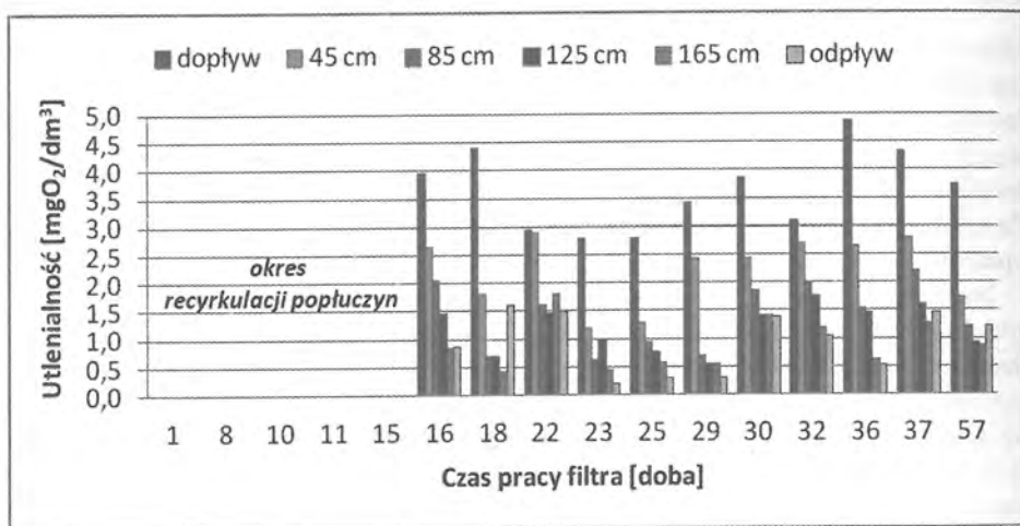
Rys. 7. Zmiana utlenialności w przekroju filtra 2 w czasie jego eksploatacji Fig. 7. Change of COD (KMnO 4 ) in a vertical section of the filter 2 during its operation.
