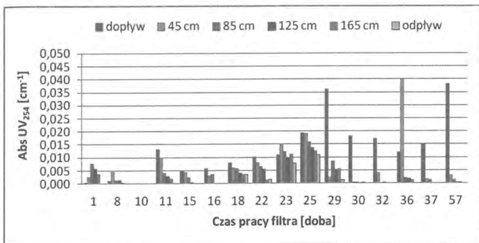
Rys. 8. Zmiana absorbancji UV254 w przekroju filtra 1 w czasie jego eksploatacji
