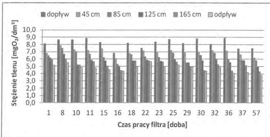
Rys. 12. Zmiana stężenia tlenu rozpuszczonego w przekroju filtra 1 w czasie jego eksploatacji Fig. 12. Change of dissolved oxygen in a vertical section of the filter 1 during its operation.
