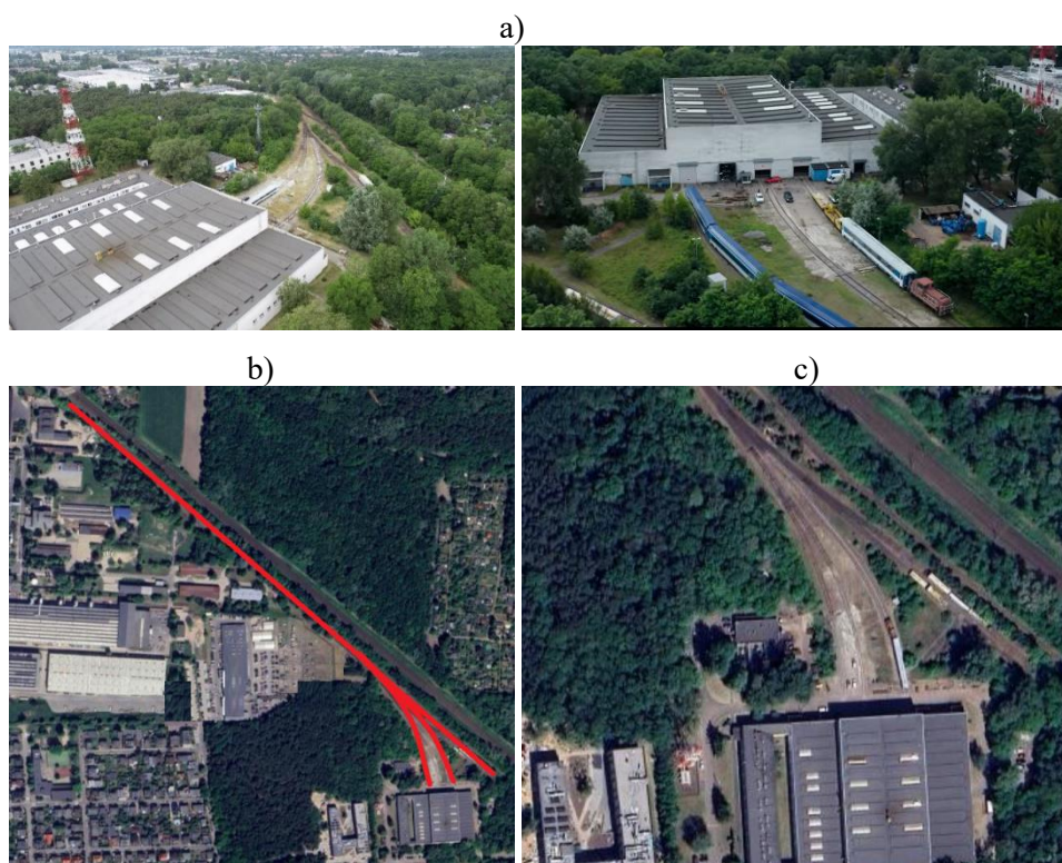
Rys. 6.9. Hala oraz bocznica kolejowa przy Ł-PIT na ul. Warszawskiej 181 w Poznaniu: a) widok na halę, b) zaznaczone tory na bocznicy, c) widok na bocznice w pobliżu hali
