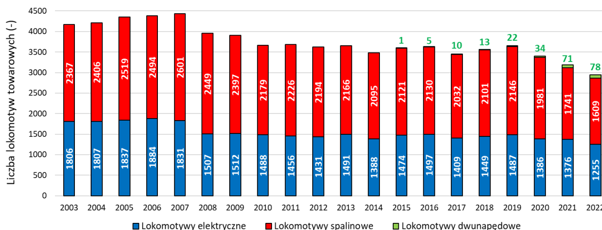
Rys. 2.16. Ilostan lokomotyw towarowych w Polsce w latach 2003-2022 (na podstawie [37])
