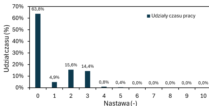
Rys. 4.11. Histogram obciążeń silnika spalinowego lokomotywy serii SM42 pracującej na szlaku (modernizacja linii - prace budowlane) [100]
