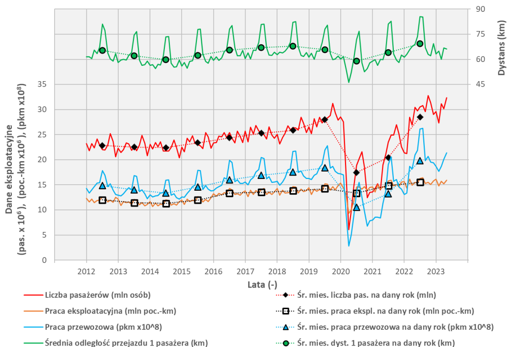
Rys. 2.4. Szczegółowe dane miesięczne oraz średnie miesięczne dla danego roku dla kolejowych przewozów pasażerskich w Polsce na przestrzeni od I.2012 do V.2023 (na podstawie [37,43])
